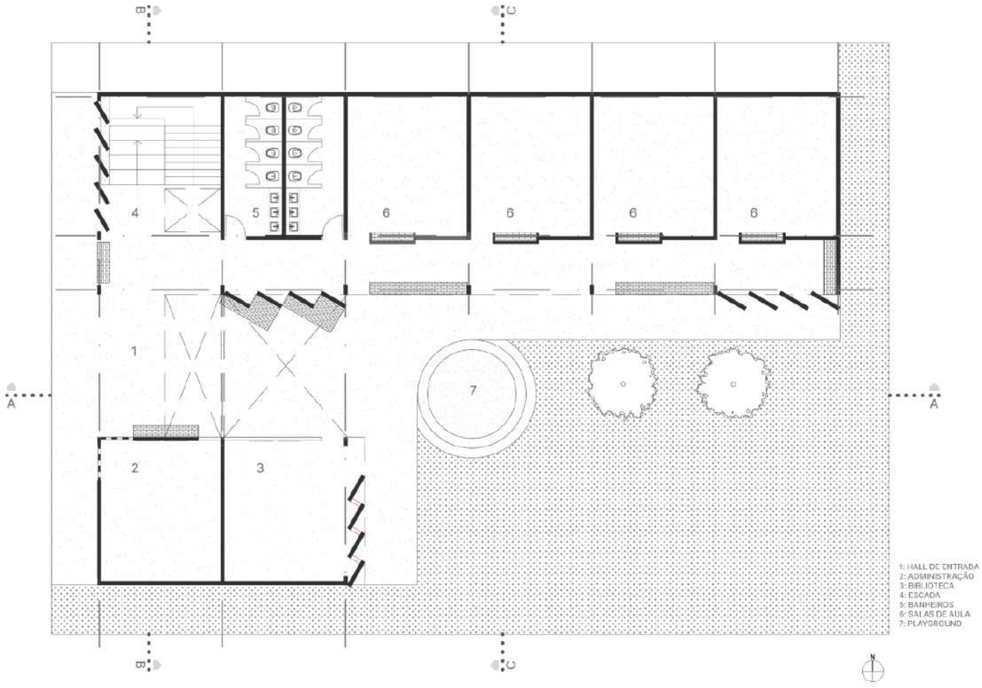
PLANTA PAVIMENTO TÉRREO
